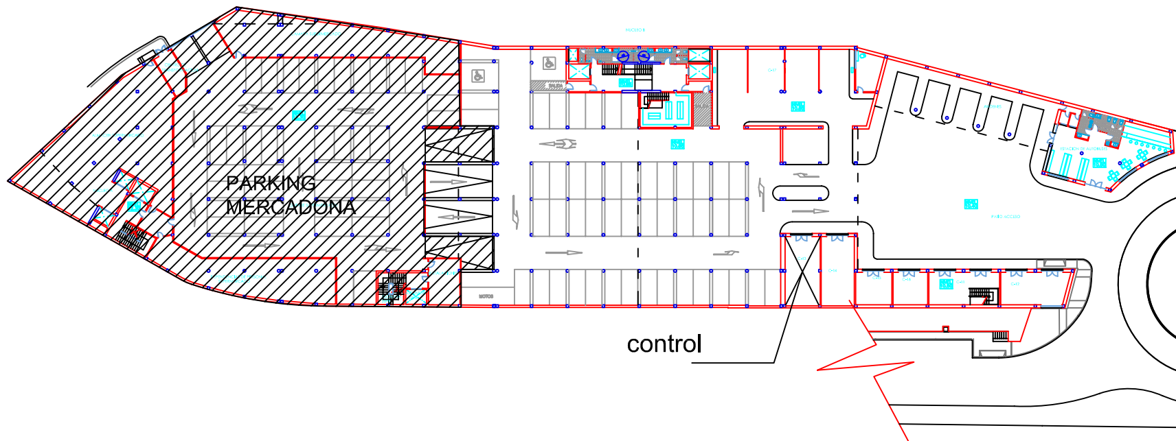
PLANTA -1 (ACCESO RODADO)
